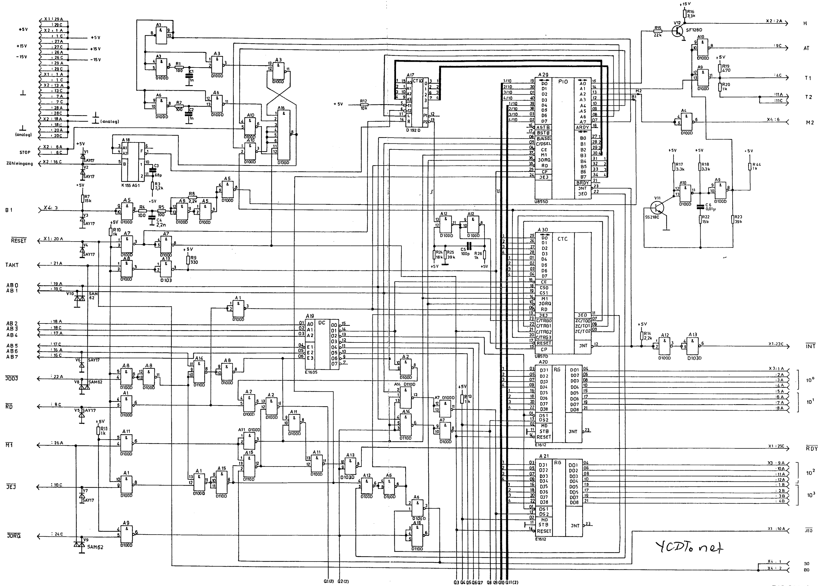
Stromlaufplan Электрическая схема Wiring Diagram
